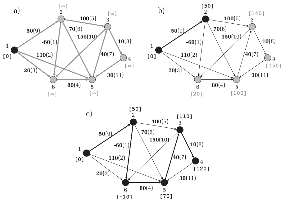
6.3. ábra. Bellman–Ford-stratégia
